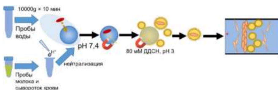
Рис. Схема мТФМЭ антибиотиков из реальных объектов с последующим определением методом КЗЭ-УФ.
