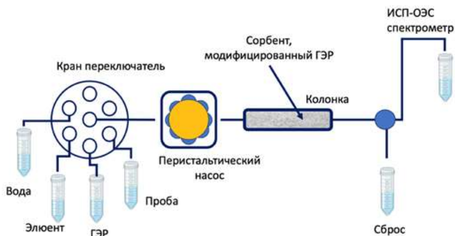
Рис. Гидравлическая схема для автоматизированного определения тяжелых металлов в пищевых продуктах методом ОЭС-ИСП
